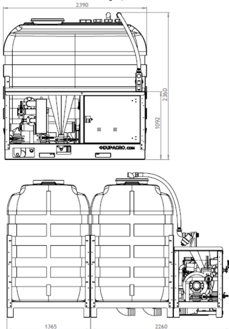
M5D-S4-2M Dubbel tank afmetingen; 2390x3625x2360mm
