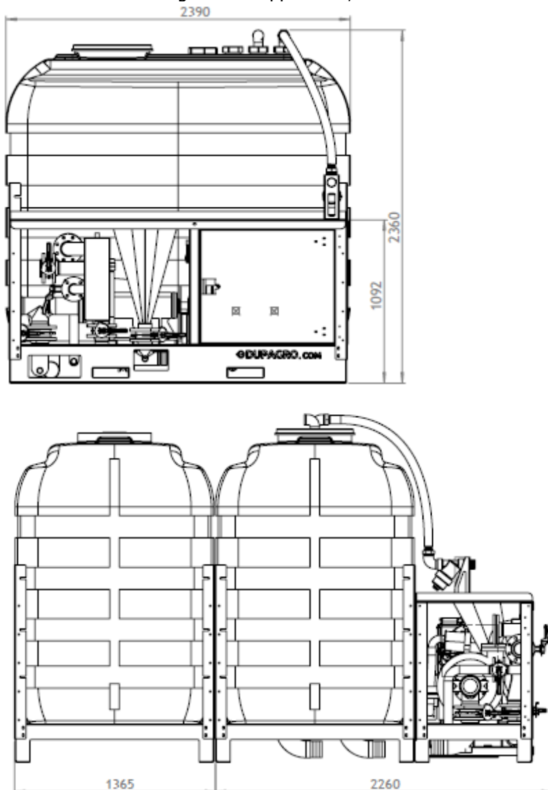
M5D-S4-2M Abmessungen des Doppeltanks; 2390x3625x2360mm
