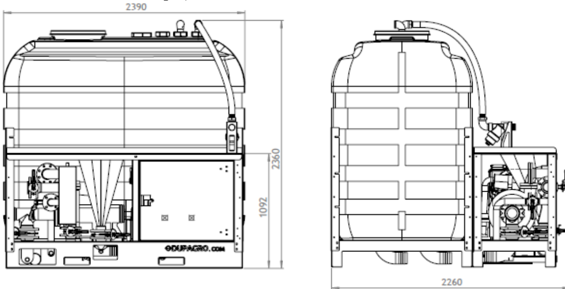
M5D-S4 Einzeltankabmessungen; 2390x2260x2360mm
