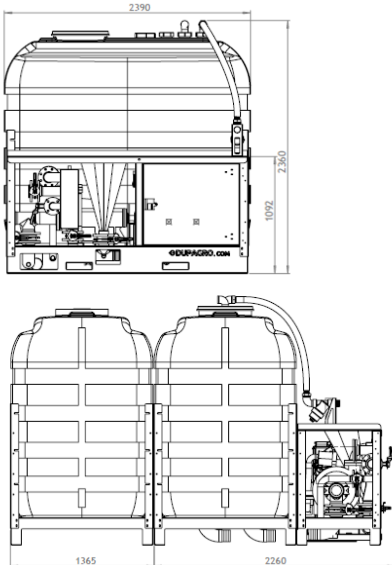
M5E-S4-2M Abmessungen des Doppel tanks; 2390x3625x2360mm
