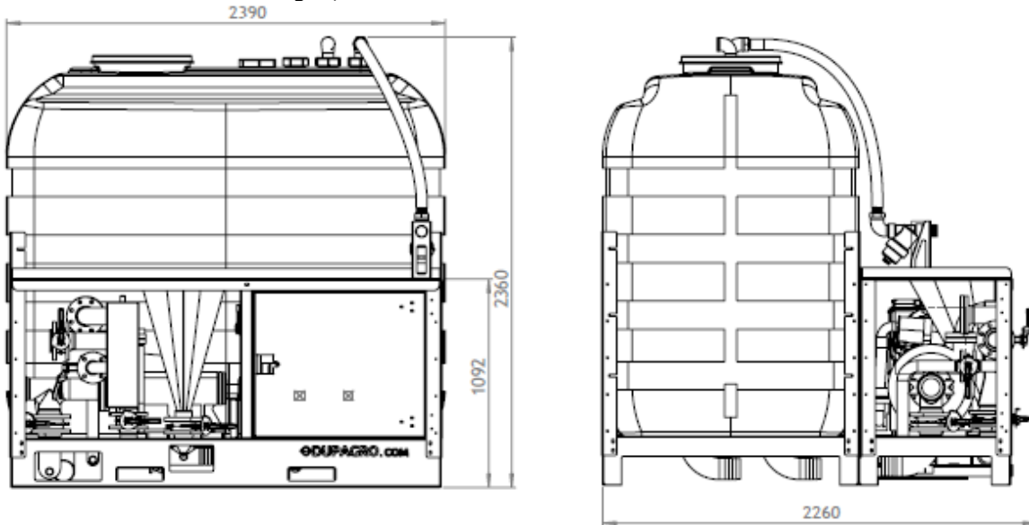
M5E-S4 Einzeltankabmessungen; 2390x2260x2360mm
