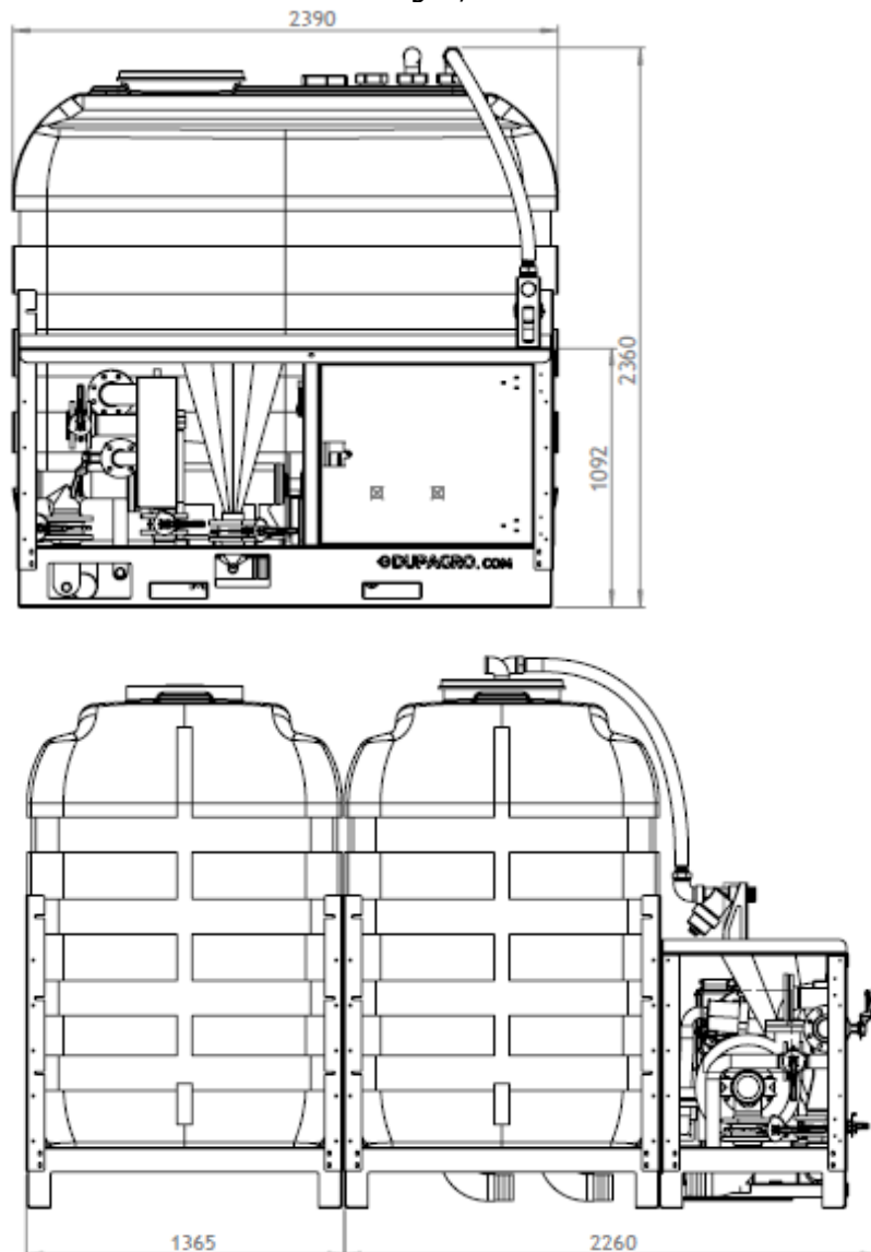
M5E-S4-2M Dubbel tank afmetingen; 2390x3625x2360mm
